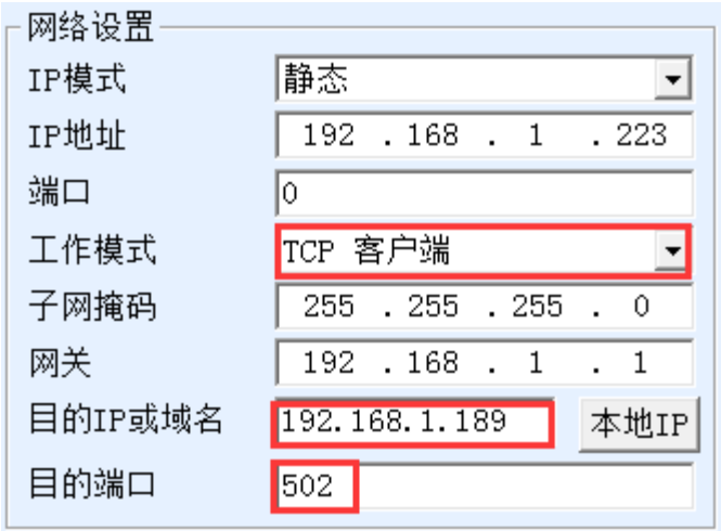
图 23Modbus TCP 做客户端。
