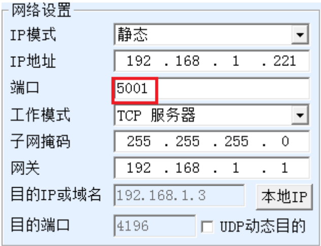
图 30 既做客户端也做服务器
