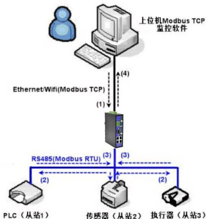
图 51 存储型 Modbus 网关工作方式
