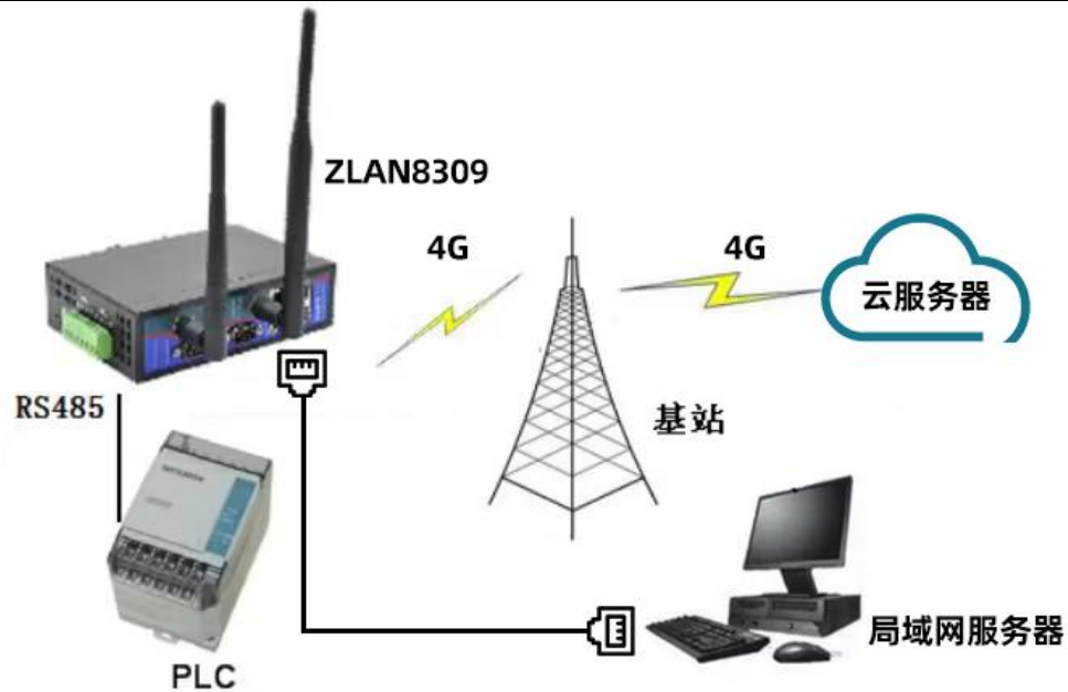
图 2 连接示意图
