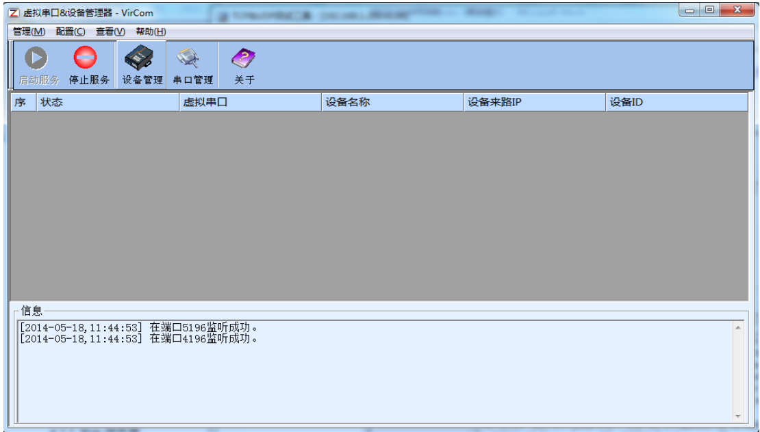
图 7 ZLVircom 主界面
